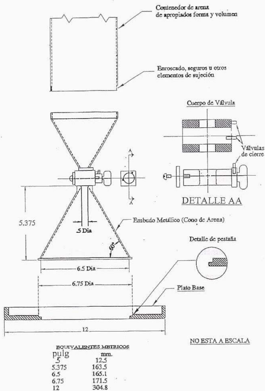
FIG. 1 APARATO DE DENSIDAD
